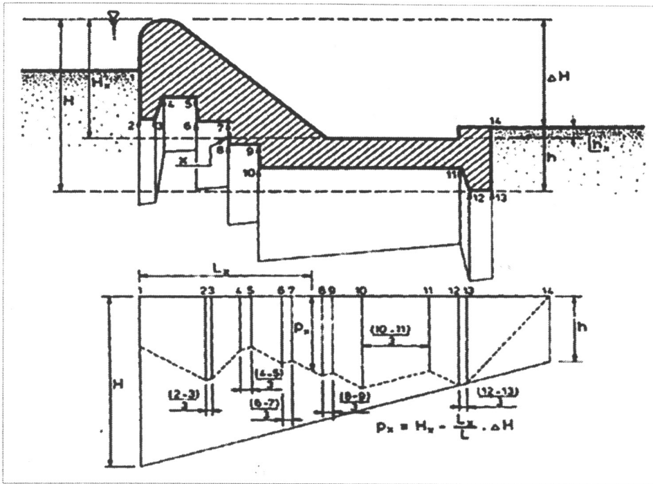
Gambar 3-12. Gaya Tekan ke Atas pada Pondasi Bendung
