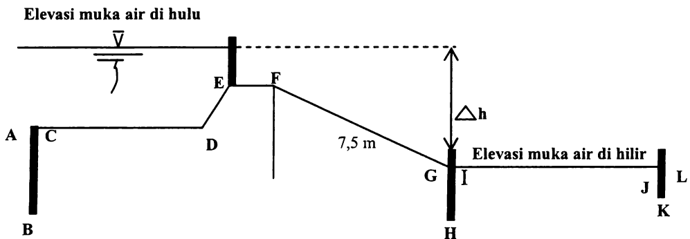
Gambar 3-13. Panjang Creep Line Sesuai Metode Bligh
