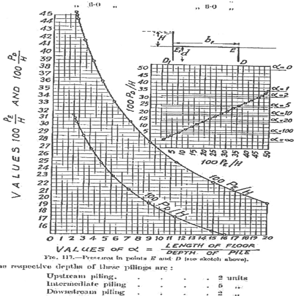
Gambar 3-15. Grafik Khosla's Secara Empiris
