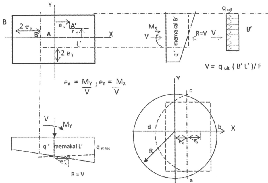
Gambar 2-4. Metode Menghitung Ukuran Telapak Efektif
