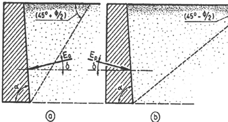
Gambar 3-6. Tekanan (a) Aktif dan (b) Pasif, Menurut Rankine
