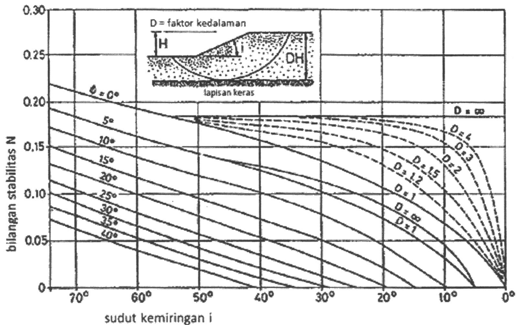
Gambar 2-1. Kurve-Kurve Taylor untuk Stabilitas Tanggul (dan Capper, 1976)
