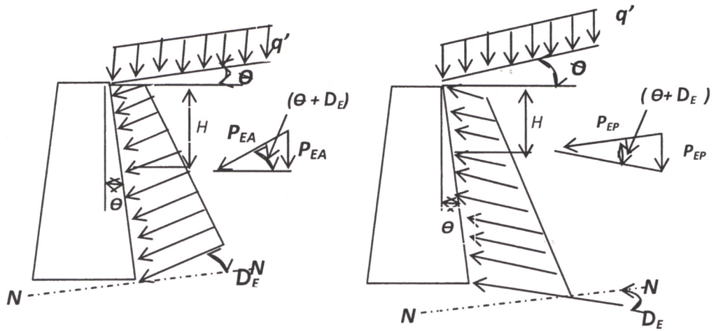
Gambar 3-26. Tekanan Tanah Akibat Gempa
