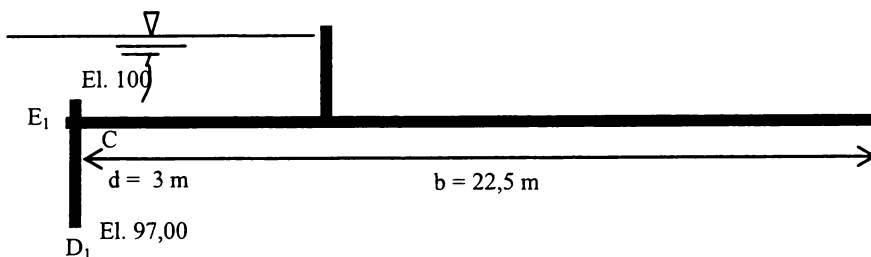
Gambar 3-22. Hydraulic Structures tentang Penggunaan Grafik Khosla dengan Asumsi SheetPile di Hulu
