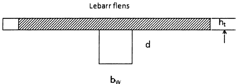
Gambar 5-9. Balok T
