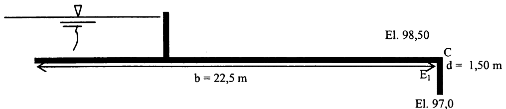
Gambar 3-24. Penggunaan Grafik Khosla dengan Asumsi SheetPile di Hilir
