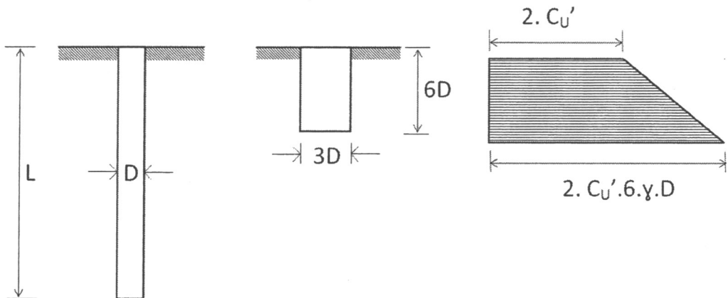
Gambar 6-4. Tahanan Lateral Tiang pada Tanah Kohesif
