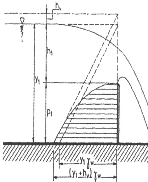
Gambar 3-9. Tekanan Hidrodinamik
