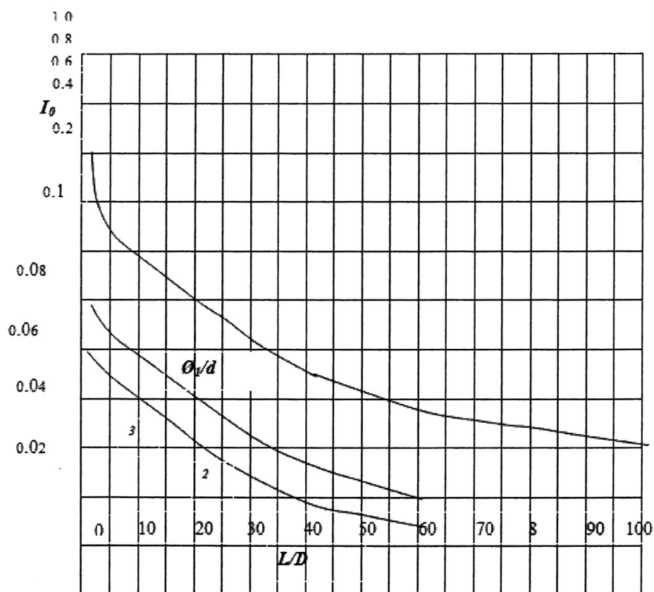
Gambar 6-14. Faktor Pengaruh Penurunan I
