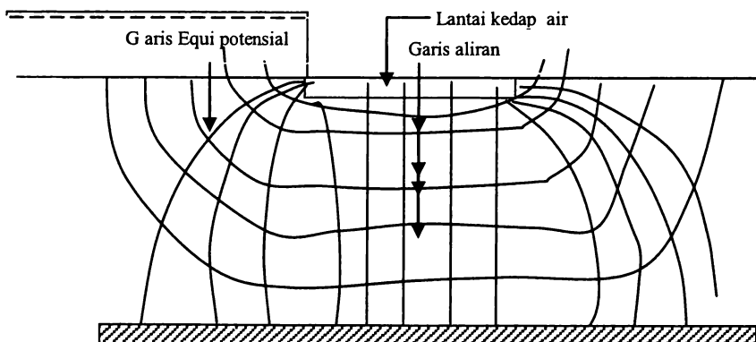
(a) Sejumlah Potensi Aliran Air Kebawah pada Sisi Terluar Sheet Pile yang Lebih Banyak daripada Permukaan Sisi dalam atau Aliran Horizontal
