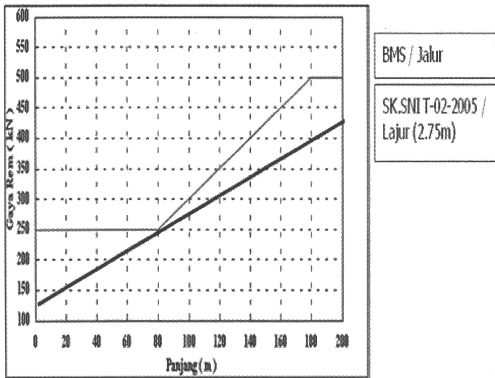
Gambar 3-2. Grafik Gaya Rem dan Panjang
