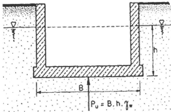
Gambar 3-8. Gaya Tekan Air ke Atas
