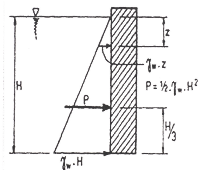
Gambar 3-7. Tekanan Air Pada Dinding Tegak
