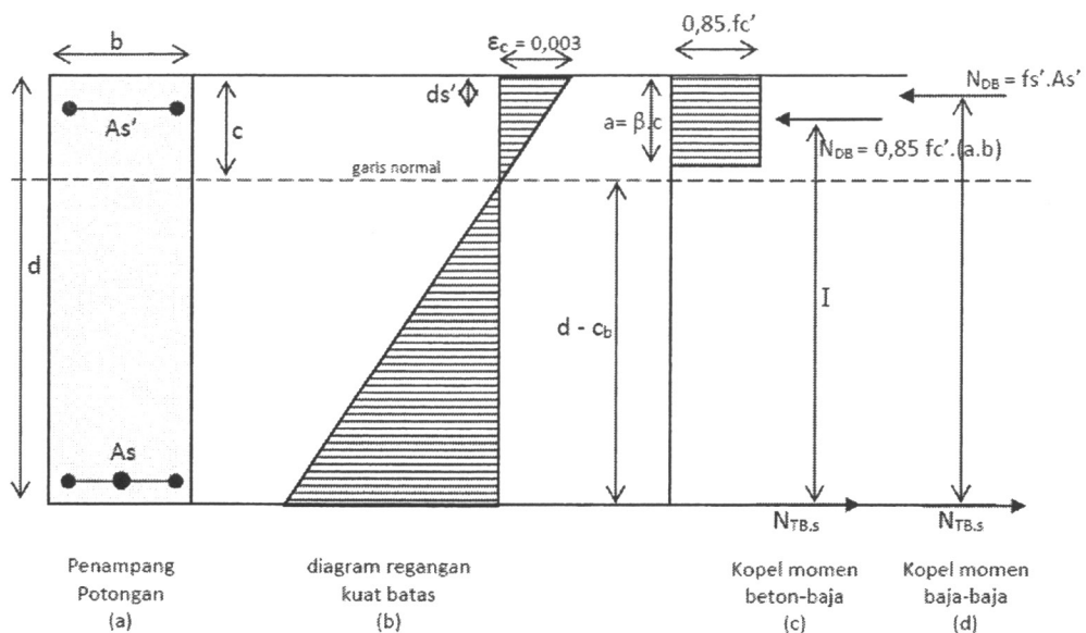
Gambar 5-5. Analisis Balok Tulangan
