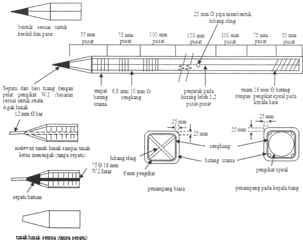
Gambar 6-19. Ujung dan Kepala Tiang
