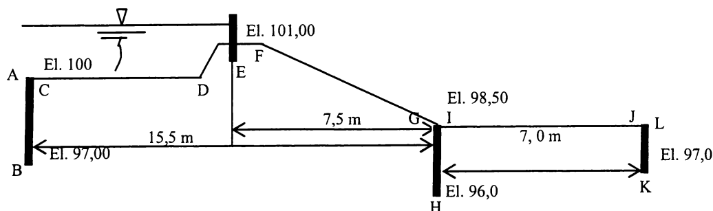
Gambar 3-21. Hydraulic Structures tentang Penggunaan Grafik Khosla
