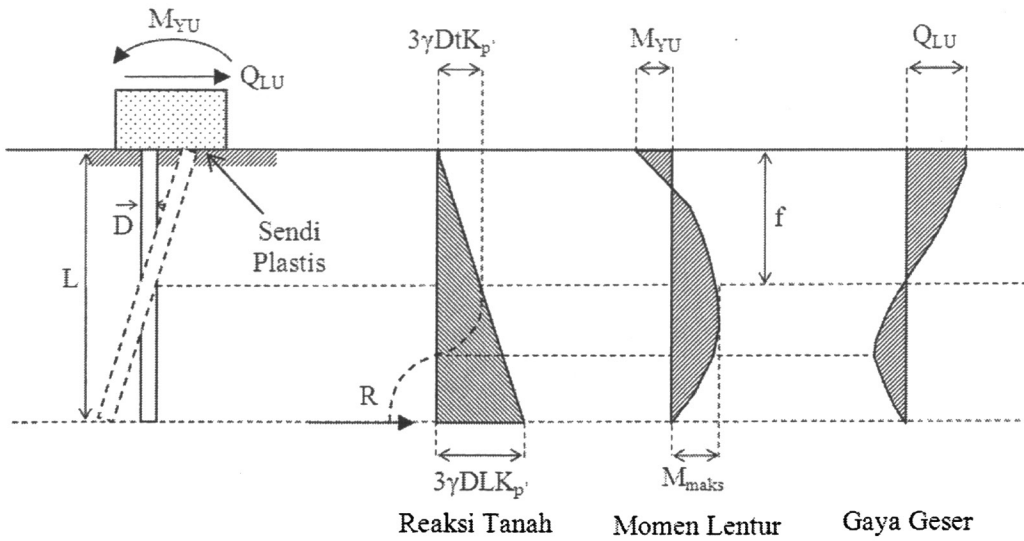
(b) Tiang Menengah Jenis Tertahan
